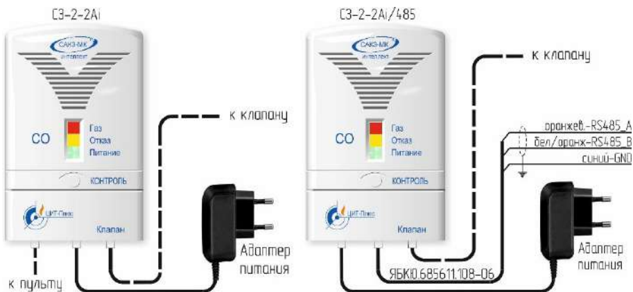
Рисунок В.1 – Типовая монтажная схема включения сигнализатора
